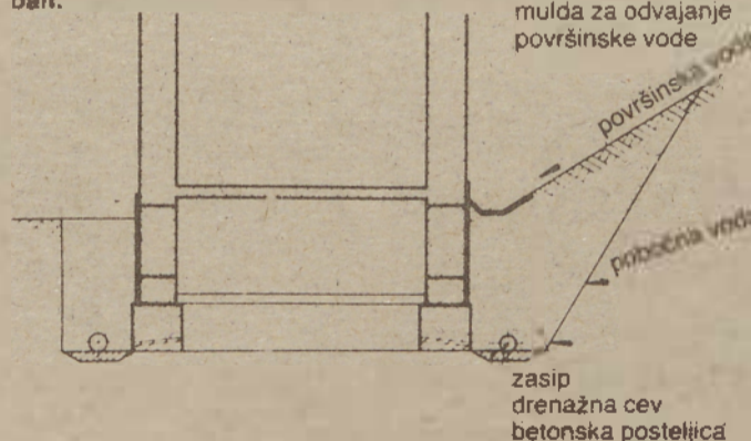
Sl. 3, primer zaščite pred pobočno vodo z drenažo pri zgradbah v nagnjenem zemljišču.
