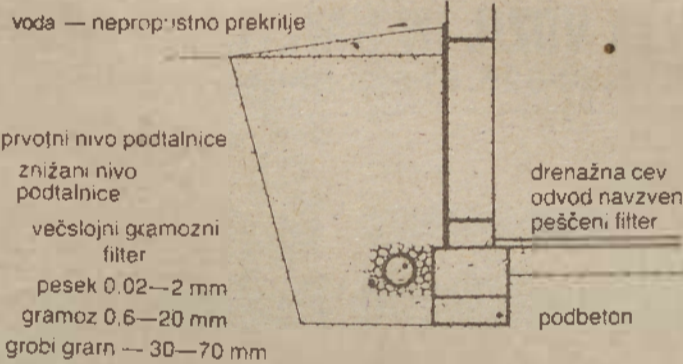
Sl. 2, primer pravilne izvedbe drenaže pri podkletnih zgradbah.
