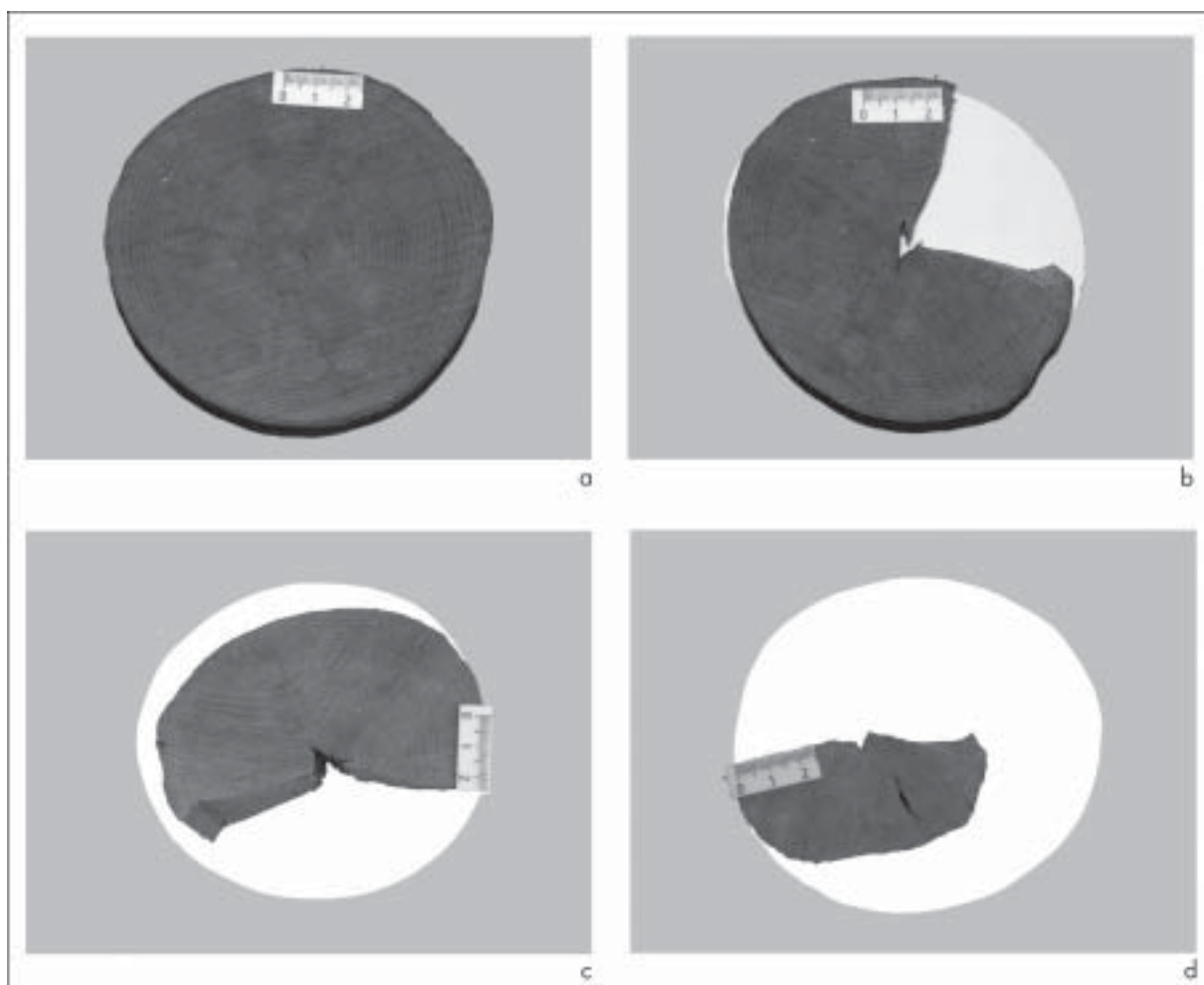
Sl. 1: Vzorec jesenovega kola, starega 4500 let, premera 12 cm in debeline 7 cm. (a) Vzorec napojen z vodo (vlažnost u = 900 \% ), (b), (c) isti vzorec med sušenjem in (d) vzorec, uravnotežen v normalni klimi (vlažnost u = 14 \% ).
