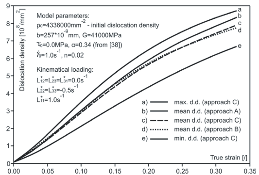
Fig. 4. Predicted dislocation density (Bergström model)
