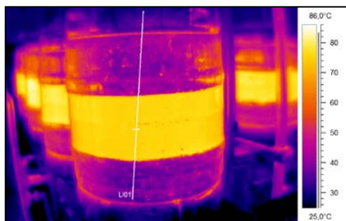
Slika 2. Poln pivski sod na polnilni liniji
