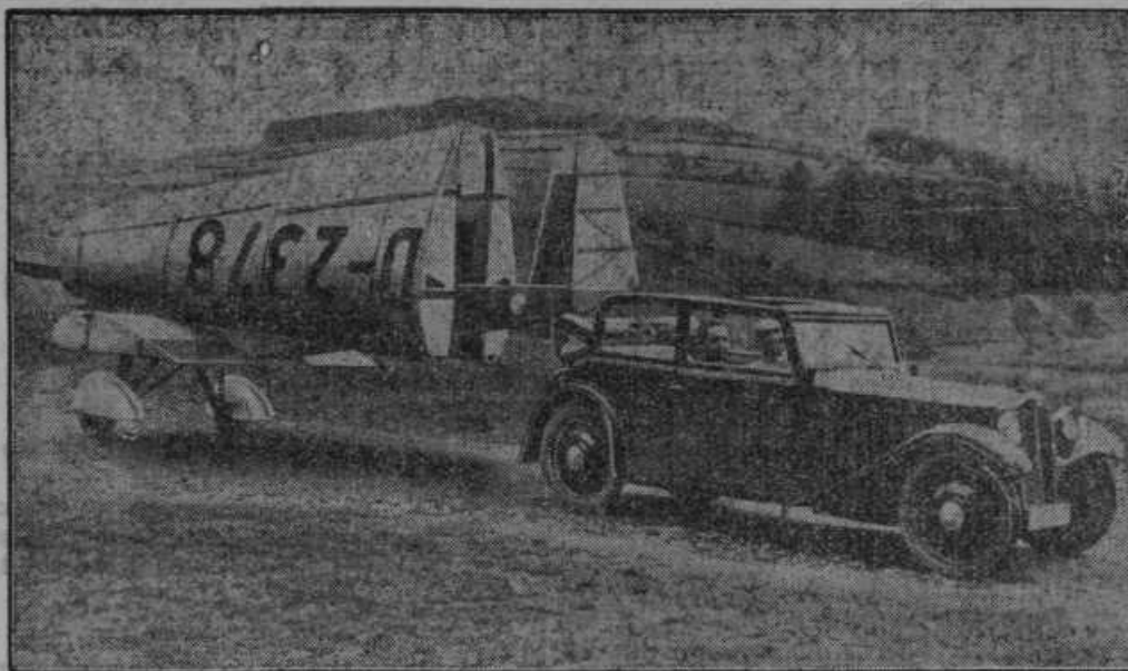
Ceno potniško letalo, ki stane 65.000 Din in vozi 105 km na uro. Večina delov je iz lesa. Slika nam predstavlja prevoz letala na letališče.
