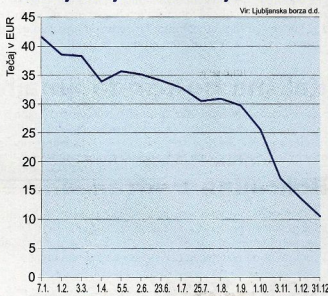
Gibanje tečajja delnic Gorenja v letu 2008
