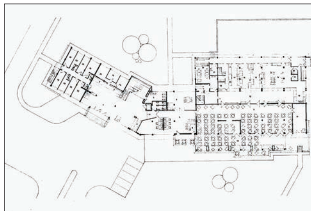
Slika 3: Hotel „Adriatik“ 1966. – Tlocrt prizemlja („Hotelski kompleks u Budvi“, 1967, 42–47).
