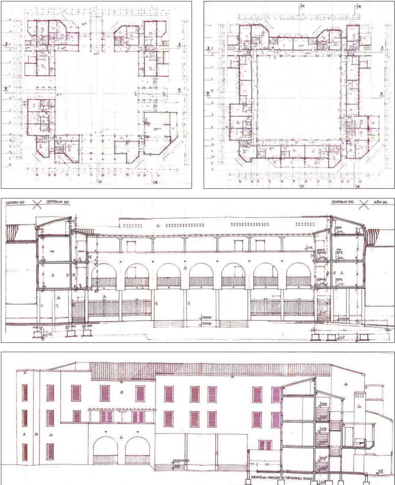
Slika 13: Trg čempresa, centralni dio – Tlocrt prizemlja i prvog kata; Presjek kroz unutrašnje dvorište i južna fasada (DACG, 214.31).
