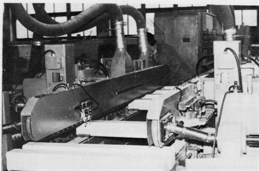
Izdelava podnožij v obratu pohištva
