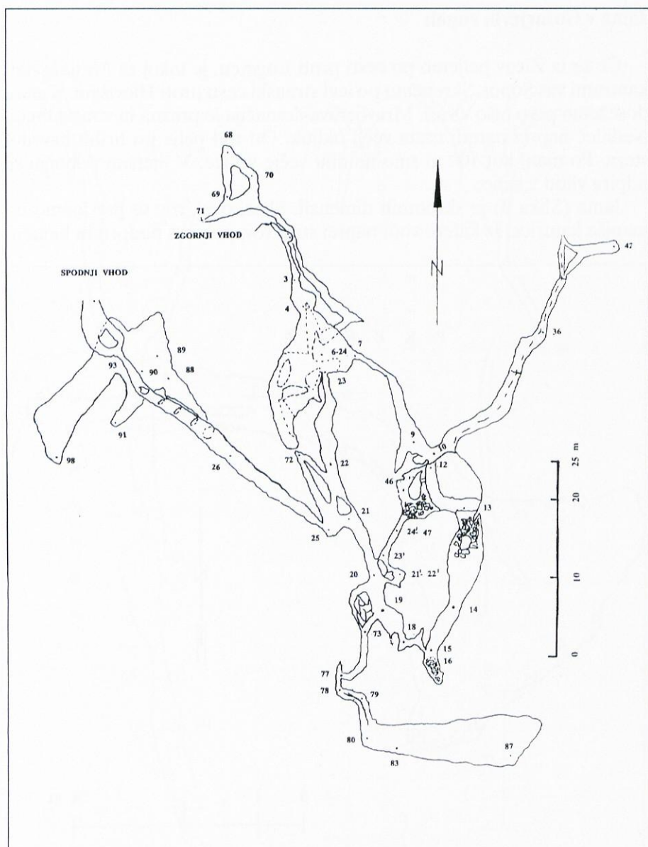
Slika 4: Načrt Mravljetovega brezna v Gošarjevih rupah (Marko in Walter Zakrajšek, Kofler 1996)
