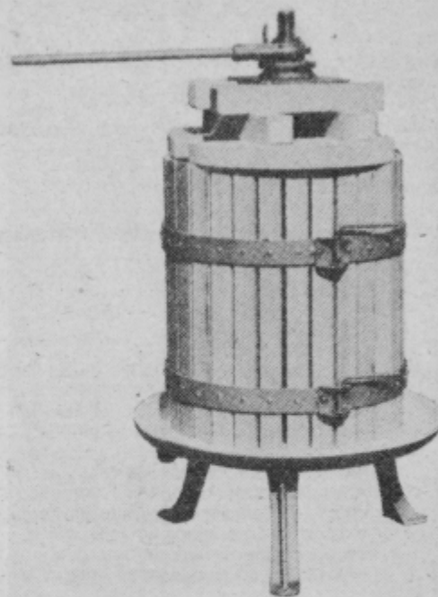
Mehanična stiskalnica TIP 25, 40, 60, 90 in 150 litrov: izdelana je iz aluminijaste skelde, leseni deli so iz bukovega lesa. Stiskanje je ročno s pomočjo račne.
