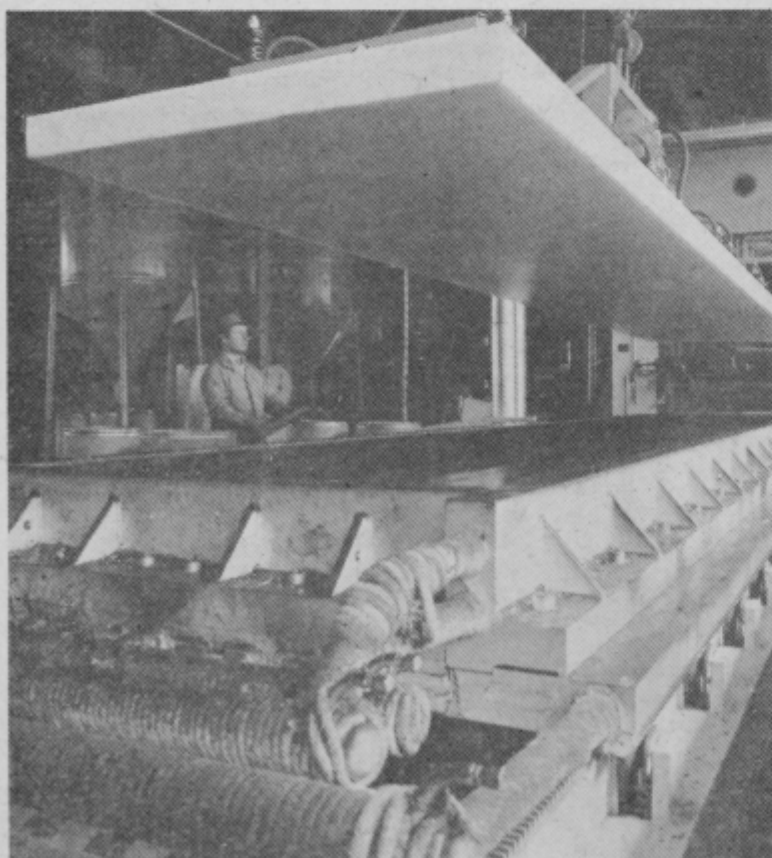
Koterm – stiskane polipropelinske plošče velikih dimenzij.
