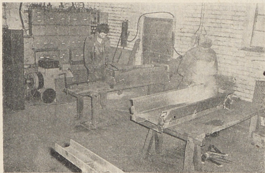
Izdelovanje korit za verižne transporterje v delavnici TOZD ESD (Foto inž. T. Bregant)
