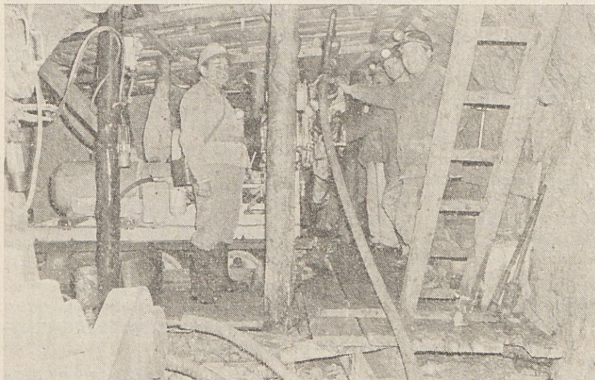
Skupina vrtalcev ZPT izdeluje vrtino H j -3/73, z vrtalnim strojem Longyear 34, na zvezni proggi med Hrastnikom in Dolom (Foto inž. T. Bregant)
