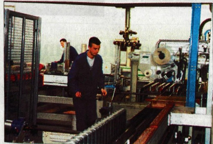
V industriji pohištva Alpes, d.d., danes pri obdelavi treh vlačilcev ivernih plošč na dan uporabljajo računalniško krmiljene stroje.
