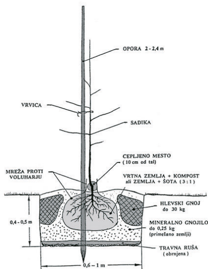
Shema sadilne jame
