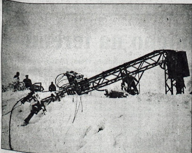
Ledenemu oklepu in teži žledu so klonili vodniki, konzole, izolatorji, drogovci in tudi jekleni jambor transformatorske postaje na Kovskem vrhu.
