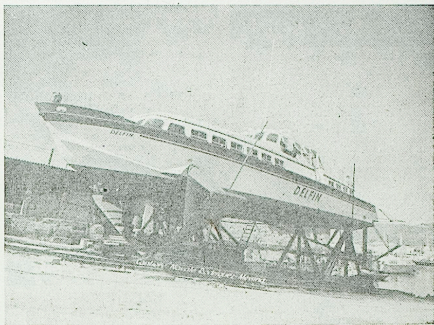
Potniški hidrogliser »Delfin«, ki ga je za avtoturistično podjetje Slavnik v Koprju izdelala ladjedelnica Rodriguez v Messini na Siciliji (na sliki), je minuli ponedeljek popoldne prispel v Koper, kjer ga je na pomolu sprejela množica radovednih meščanov
