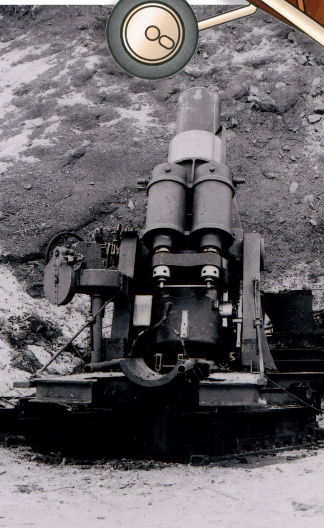
Škodin možnar, kal. 30,5, na vojni liniji
