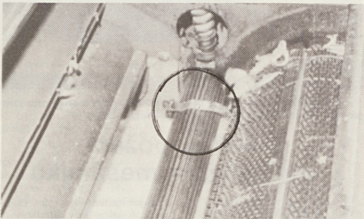
Kovinski ploščati delec je iz rahljanega dela stroja zašel k trgalnemu valju. Ob drgnjenju med bodicami valja in kovinskim delcem je nastala iskra in vnela bombažna vlakna
