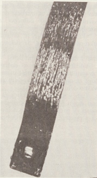
Na kovinskem delcu, ki je zašel med igle trgalnega valja, so vidne praske, ki so jih povzročile le-te. Ob tem so nastale iskre, ki so vnele bombažna vlakna.
