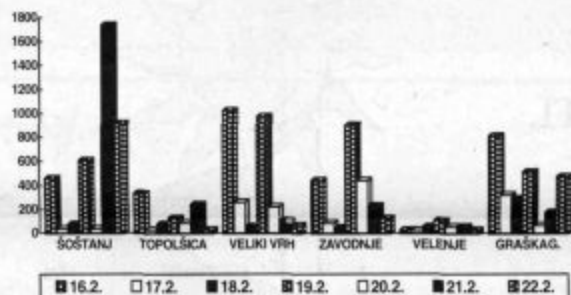
MAKSIMALNE POLURNE KONCENTRACIJE SO 2 od 16. februarja do 22. februarja 1998
