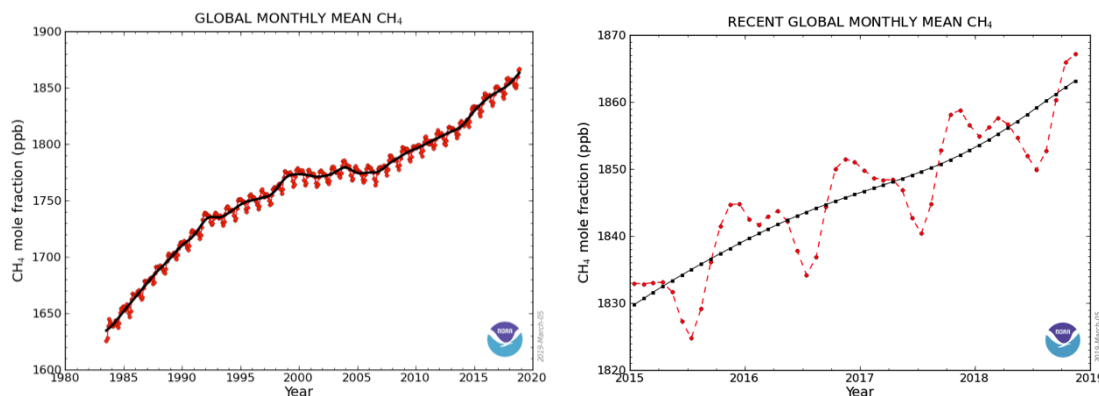
Slika 1: Grafa prikazujeta povprečno mesečno koncentracijo metana (CH 4 ) za obdobji 1980–2019 in 2015–2019 [14]. Koncentracija metana je izražena v enotah delcev na milijardo delcev (ppb). Na grafu, ki prikazuje krajše časovno obdobje, so opazna letna nihanja koncentracije.
