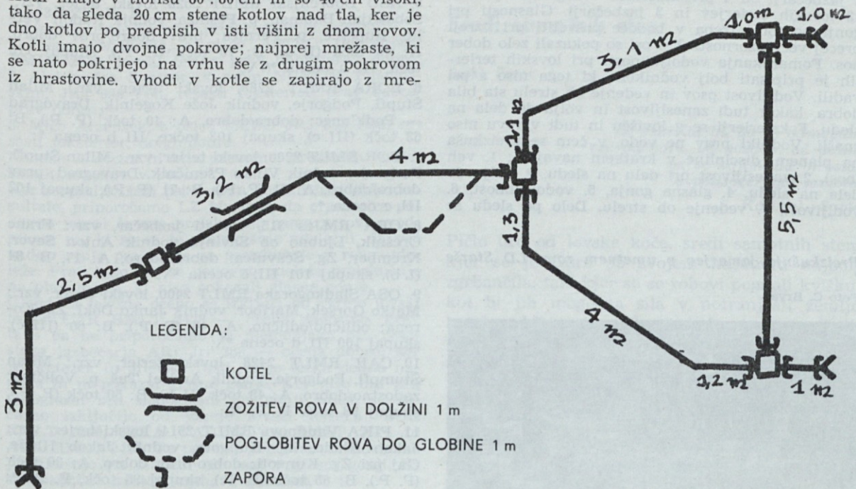
Tloris umetnega rova LD Starše
