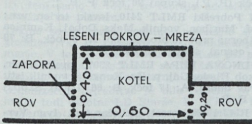
Podolžni prerez kotla
