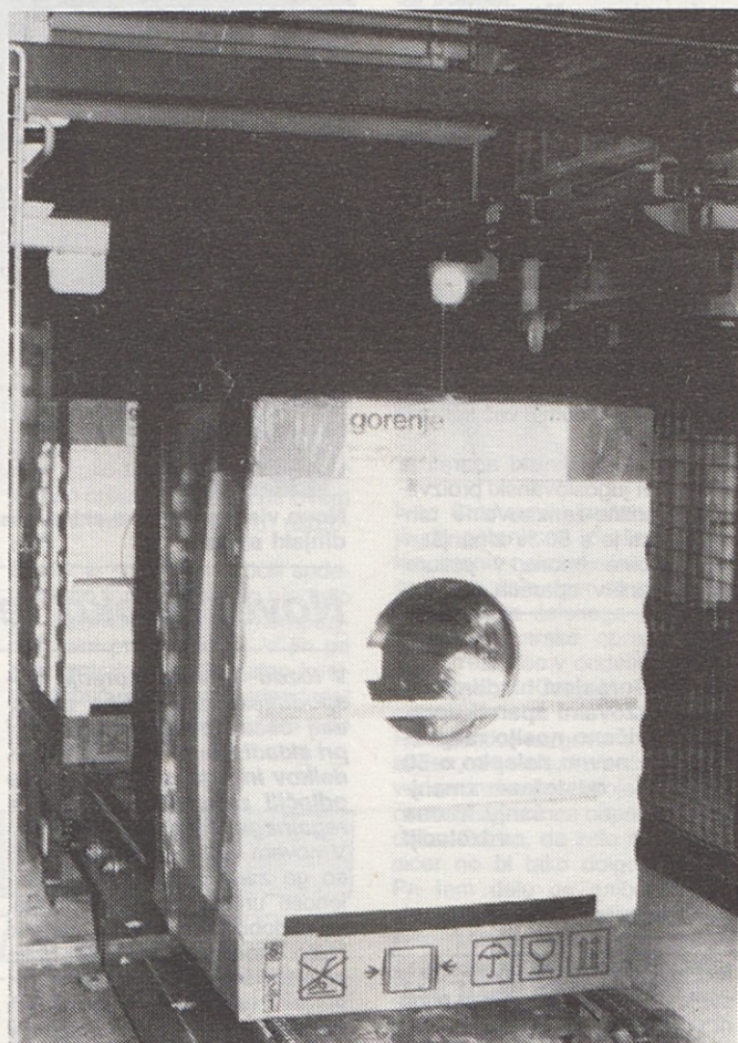
Od prejšnjega tedna naprej prihajajo s tekočih trakov pralni stroji v novi embalaži. Gre za novo embaliranje s toplotno skrčljivo folijo, ki jo segrevajo z zemeljskim plinom, kar je novost za celotno Gorenje.
