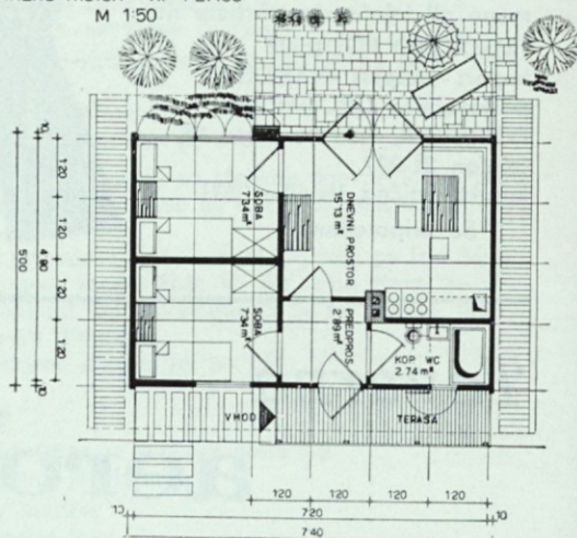
VIKEND HIŠICA TIP PL/100 M 1:50
