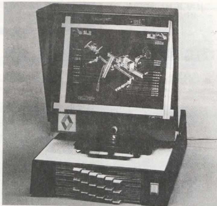
Čitalec mikrofilma (kartice) za servisno službo in rezervne dele.
