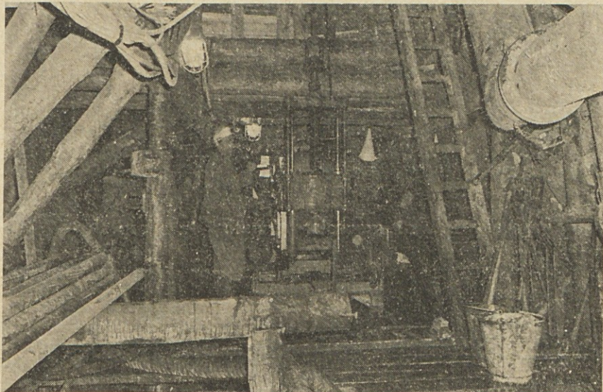
Vrtalna garnitura J-600 pri vrtanju vrtine Oj—1/77, v jami Ojstro, na V. obzorju. Garnituri streže Stane Lipeč. (Foto A. Bregant)
