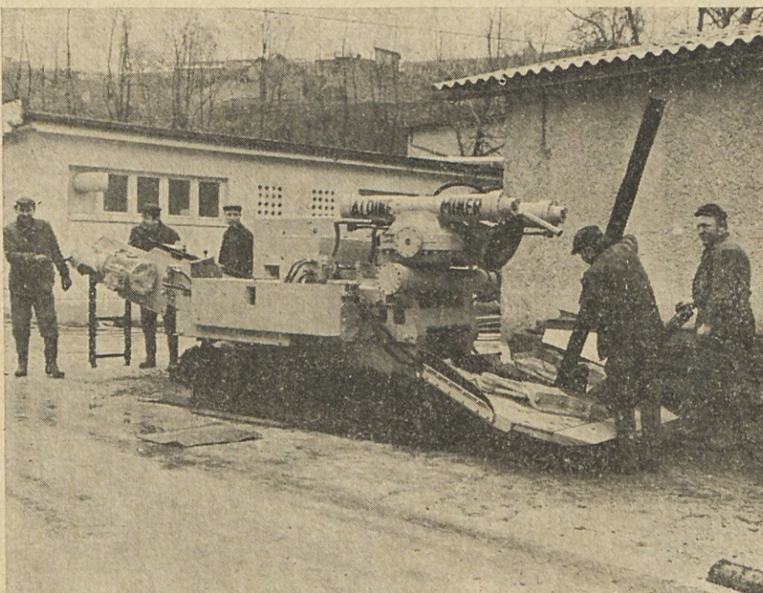
TOZD Rudnik premoga Trbovlje je prejela nov stroj za izkopavanje jamskih prog — Alpine Miner F6A, ki ga je dobavila firma Vöest — Alpine, Werk Zeitweg, Avstrija. Fotografija kaže montažo stroja na dvorišču RPT. (Foto A. Bregant)
