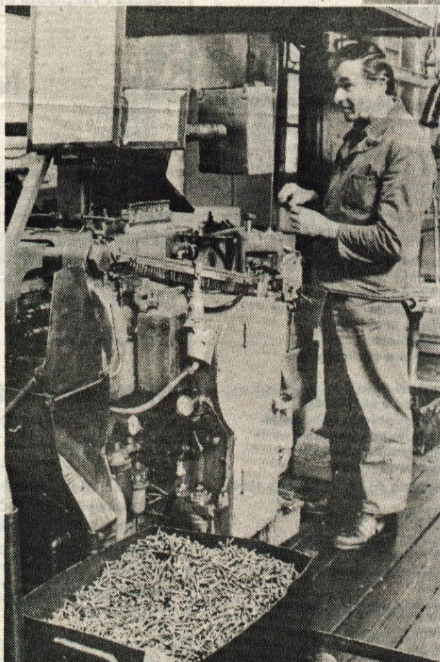
Delo pri večudarni stiskalnici za izdelavo vijakov in odkovkov
