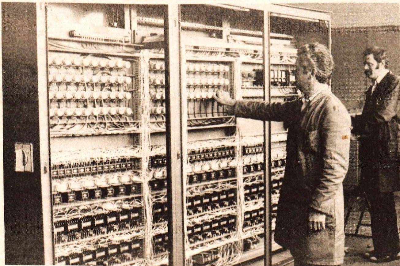
Stikalna omarica izdelana v Instalacijah. – Foto: F. Perdan
