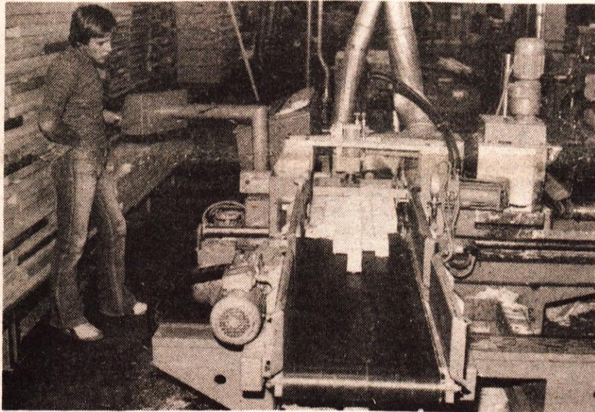
Priprava elementov za Jelovico v Alplesovem TOZD Masivne predelave. – Foto: F. Perdan
