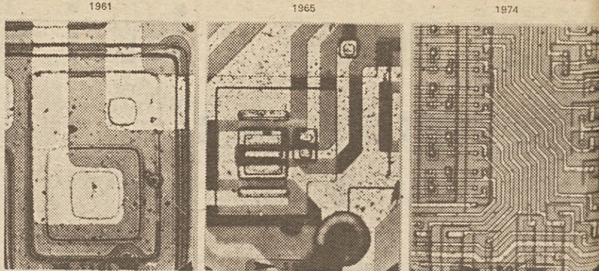
Slika 3: Fotolitografija, dimenzija vzorcev in točnost nastavitve mask (magnification=povečava).
