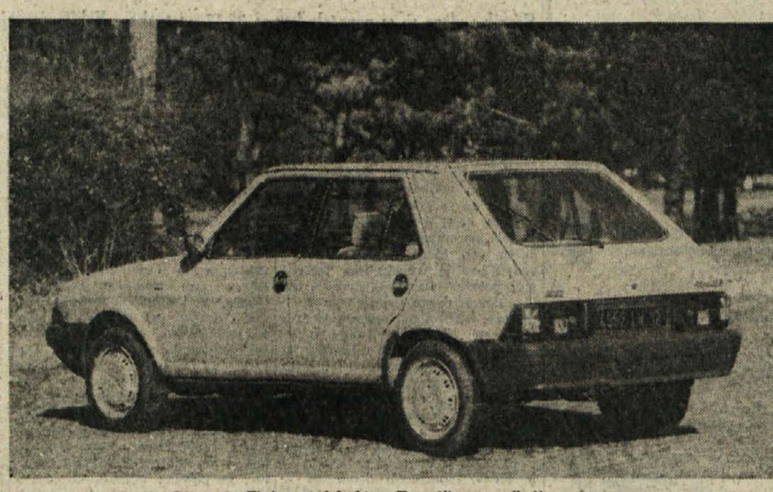
Ritmo je Fiatov model, ki v Franciji gre najbolje v acnar.
