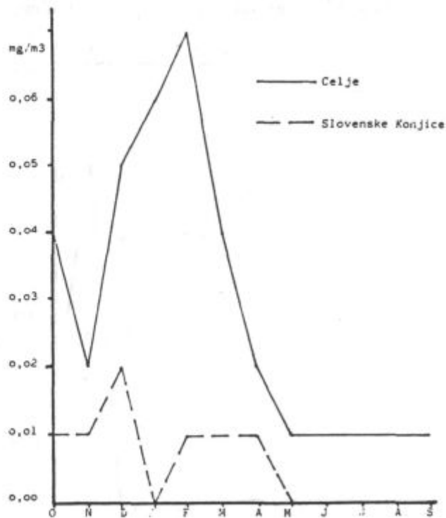
Grafikon št. 4: Gibanje povprečnih mesečnih koncentracij dima v zraku v obdobju oktober 86 — september 87 na merilnih mestih Celje — Center in Slovenske Konjice.
