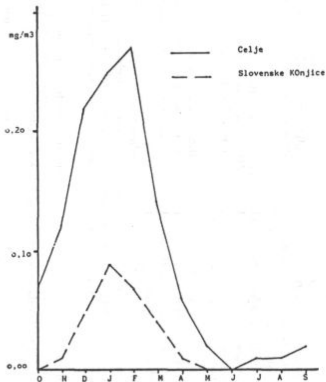
Grafikon št. 1: Gibanje povprečnih mesečnih koncentracij SO 2 v zraku v obdobju od oktobra 86 do septembra 87 na merilnih mestih Celje — Center in Slovenske Konjice.
