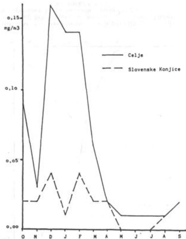
Grafikon št. 5: Onesnaženost zraka z dimom. Gibanje mesečnih vrednosti C 95 v obdobju oktober 86 – september 87 na merilnih mestih Celje – Center in Slov. Konjice.
