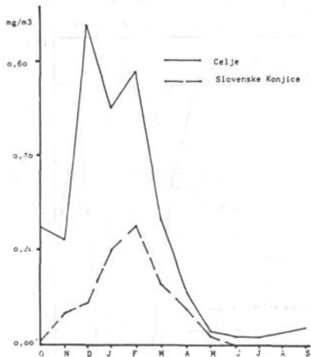
Grafikon št. 3: Gibanje maksimalnih 24-urnih povprečnih koncentracij \text{SO}_2 v zraku po mesecih, v obdobju oktober 1986 september 87 na merilnih mestih Celje — Center in Slovenske Konjice.
