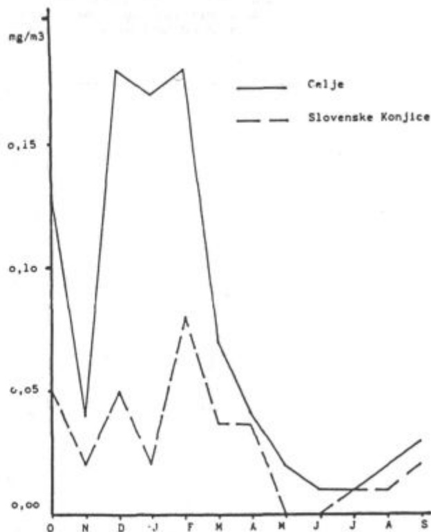
Grafikon št. 6: Gibanje maksimalnih 21-urnih povprečnih koncentracij dima v zraku po mesecih, v obdobju oktober 86 – september 87 na merilnih mestih Celje – Center in Slovenske Konjice
