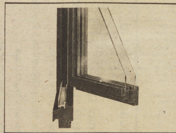
Vezano okno — prerez
