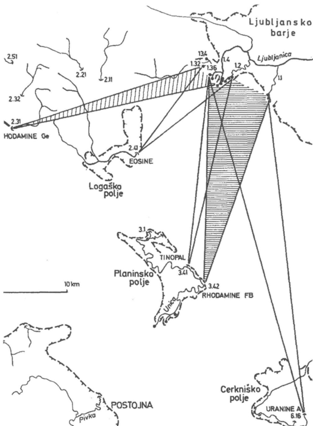
2. Razpored ugotovljenih fluorescenčnih sledil v območju poskusa (po H.Behrensu, Martina Zupan, M. Zupan: Tracing with Fluorescent Tracers. UWT, 1976, slika 59)
