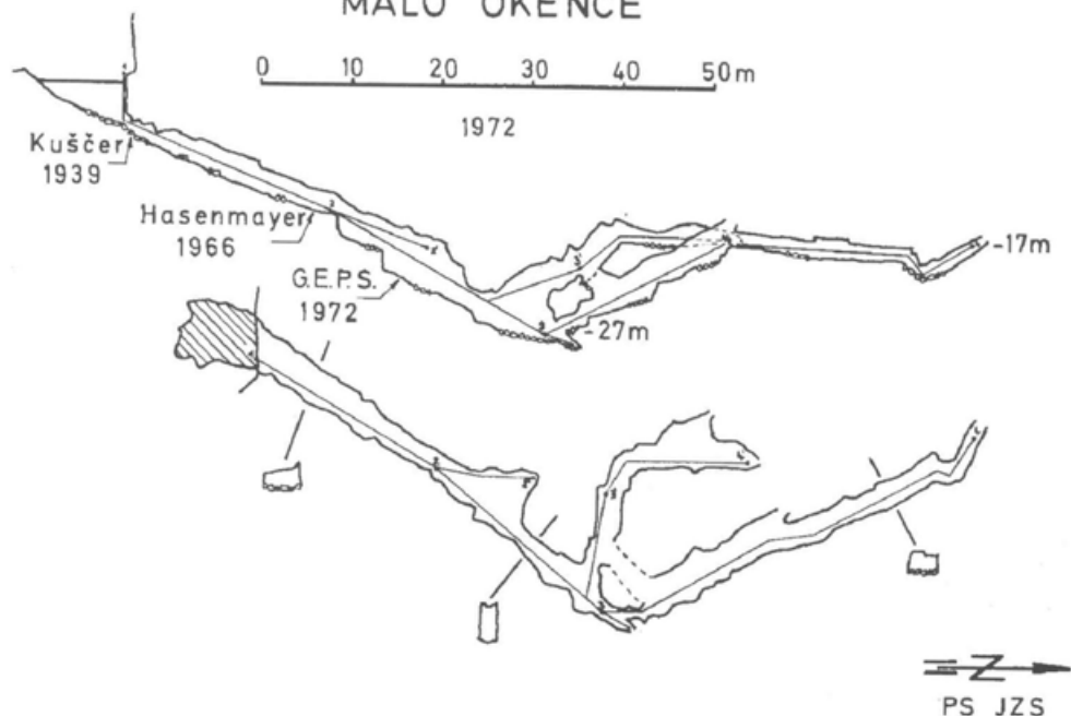
17. Malo okence, izvir Ljubljanice v Retovju, načrt raziskovanih rogov (po P.Krivicu, A.Praprotniku, Naše jame 14, 1972, slika 3)
