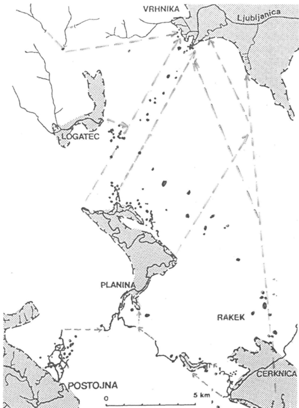
27. Kraška polja, jamski sistemi, udornice in podzemeljski tokovi v zaledju izvirov Ljubljanice med Vrhniko, Postojno in Cerknico (po P.Habiču)
