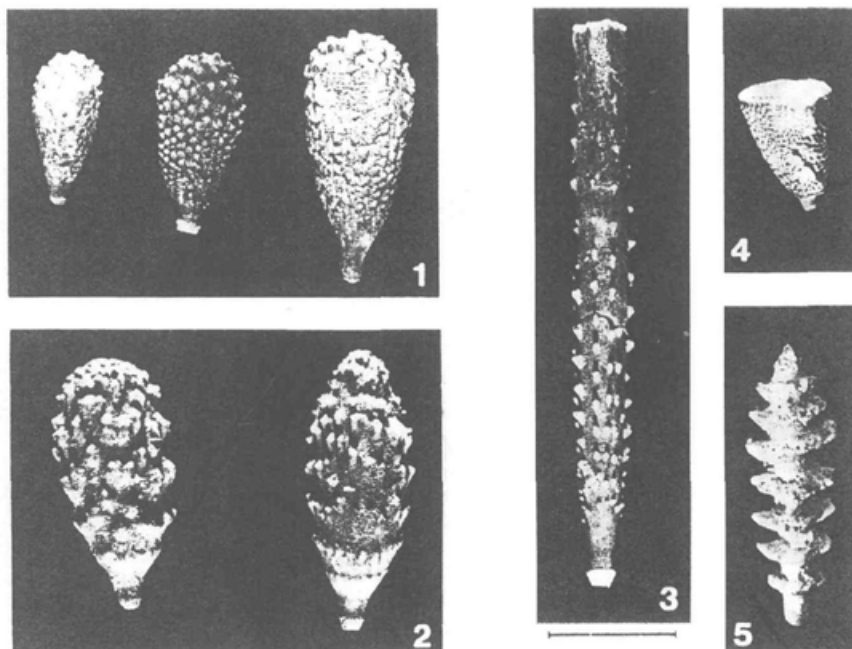
10. Ostanki triasnih morskih ježkov z Lesnega Brda. 1-5 primarne bodice vrst: (1) " Cidaris " dorsata Münster; (2) " Cidaris " sp.1; (3) " Cidaris " sp.8; (4) " Cidaris " trigona Münster; (5) " Cidaris " roemeri Wissmann.
