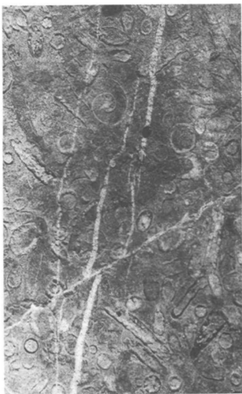
8. Črni, beložilnati zgornjepermijemski apnec na vodnjakovem pokrovu Celarjeve domačije. Zgoraj v sredini polževa hišica iz rodu Bellerophon .
