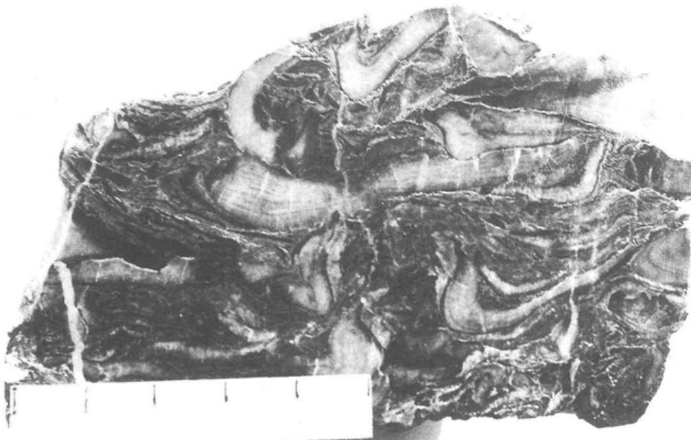
23. Litioidne in druge školjke v spodnjeljurskem apnencu pri Vrhniki
