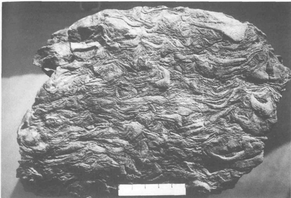
24. Nagneteni ostanki školjčnih lupin v spodnjejurskem apnencu
