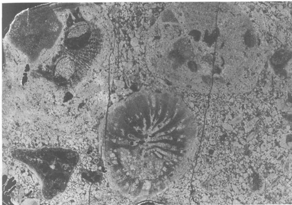
26. Oolitni in onkolitni zgornjejuški apnenec s koralami in spongijami na Logaški planoti. Foto M. Grm.
