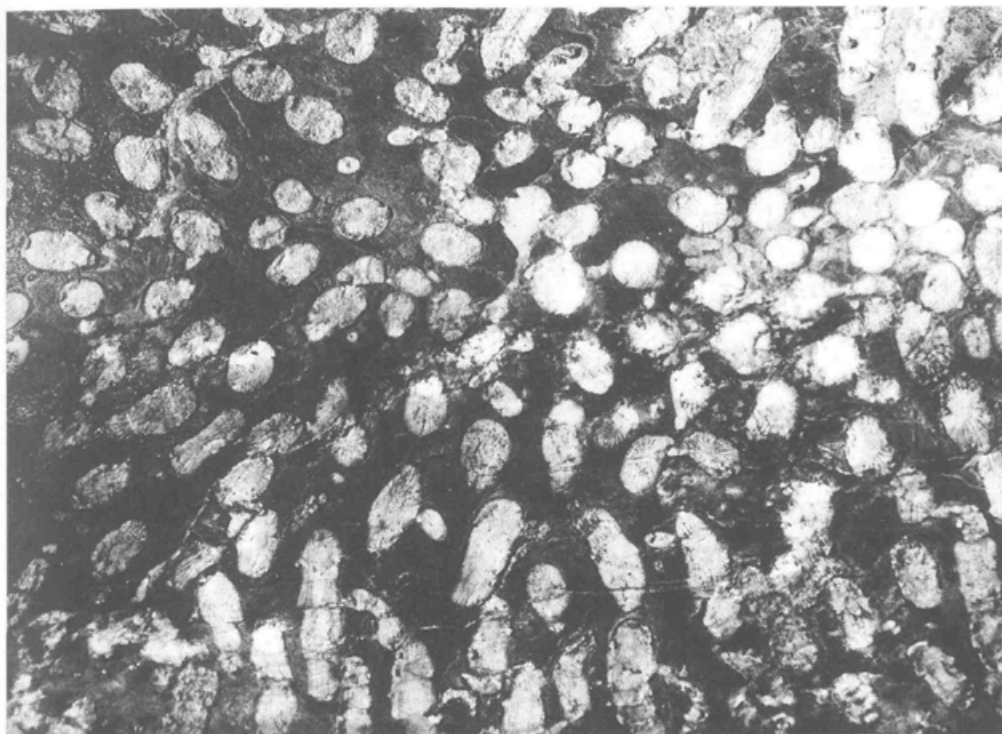
4. Koralni apnenec z vrsto Waagenophyllum indicum , zgornji permij pri Samiji
