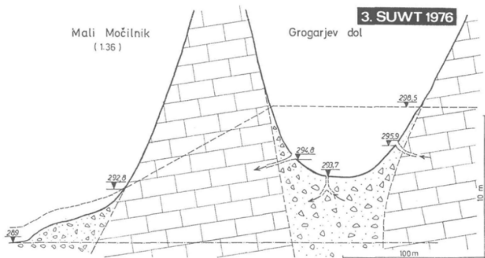
8. Presek med Malim Močilnikom in Grogarjevim dolom z najvišjo opazovano gladino kraške vode (po P.Habiču: Speleohydrological Investigations. UWT, 1976, slika 23 )
