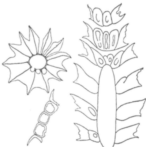
28. Shematski vzdolžni in prečni prerez apnenčeve alge Chypeina jurassica . Alga je marsikje kamnotvorna, n.pr. ob stari cesti pri tabli ponesrečenima dekletoma. Skica po M. Heraku.
