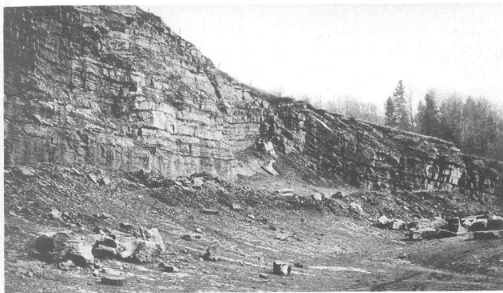
17. Črni skladnati karnijski apnenec v Mineralovem kamnolomu na Lesnem Brdu. V srednjem delu so plasti svodasto izbočene (antiklinala). Foto A. Ramovš
