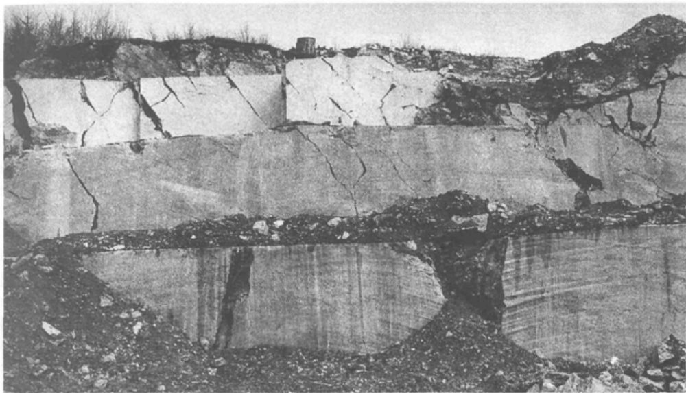
11. Mineralov kamnolom pisanega apnenca na Lesnem Brdu. V kamnini je vse polno razpok, ob katerih je voda izjedla manjše in večje zajede, prostore in celo jame. Foto A. Ramovš
