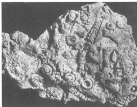
15. Zelena apnenčeva alga Diplopora annulata , kamnotvorna v zgornjetriasnem cordevolskem apnencu pri Borovnici. Leg. A. Ramovš, foto V. Finžgar
