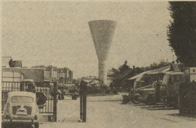
SOBOŠKI ZBIRALNIK VODE — Prostornina zbiralnika, ki ga je možno videti že od daleč, je 600 kubičnih metrov, zmogljivost črpališča pa je 50 sekundnih litrov. Foto: M. Jerše.
