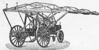
Dvokolesne in štirikolesne premikalne lestve.
