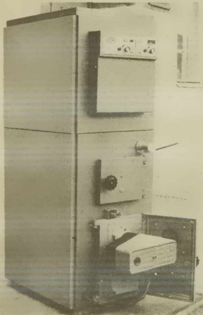
MODEL UL – Univerzalni toplovodni kotel z ali brez bojlerja za ogrevanje sanitarne vode. Možnost uporabe tekočih, plinastih in trdih goriv.
