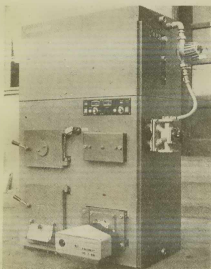
MODEL KL – Kotel z dvojnimi kuriščem z ali brez bojlerja, združuje dva kotla v enem. Eno kurišče je namenjeno za uporabo olja in plina in drugo za kurjenje trdih goriv.
