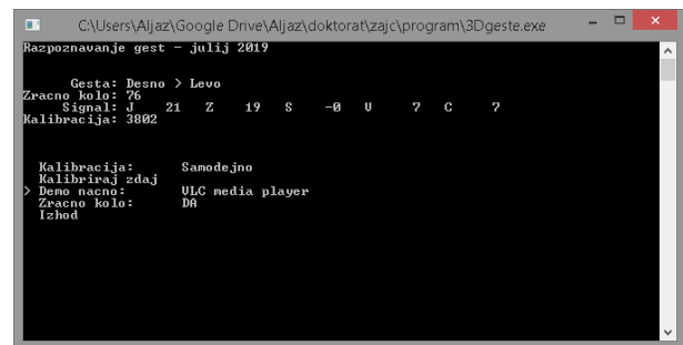
Slika 7: Izgled programa za upravljanje z gestami.
