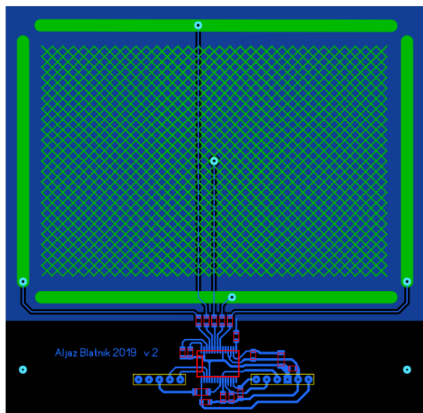
Slika 2: Končni izgled dvoslojne tiskanine senzorja.
