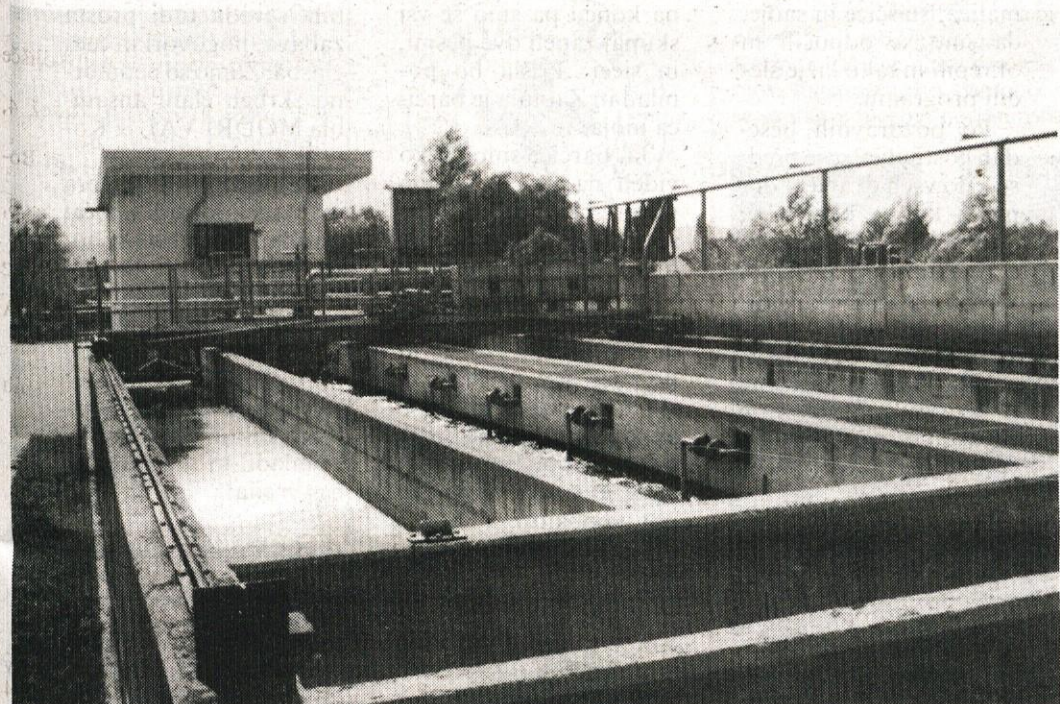
Vrhnika čistilna naprava, kjer deluje samo mehanično čiščenje vode.
