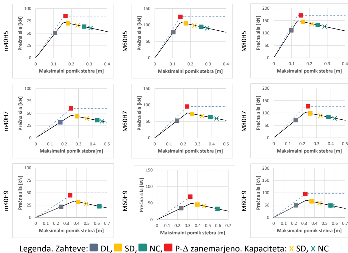
Slika 6. Rezultati N2-metode za šibkejši od dveh upoštevanih potresnih vplivov ( S_\beta = 0,394 g): polna črta – upoštevani P-Δ učinki; črtkana črta – zanemarjeni P-Δ učinki.
