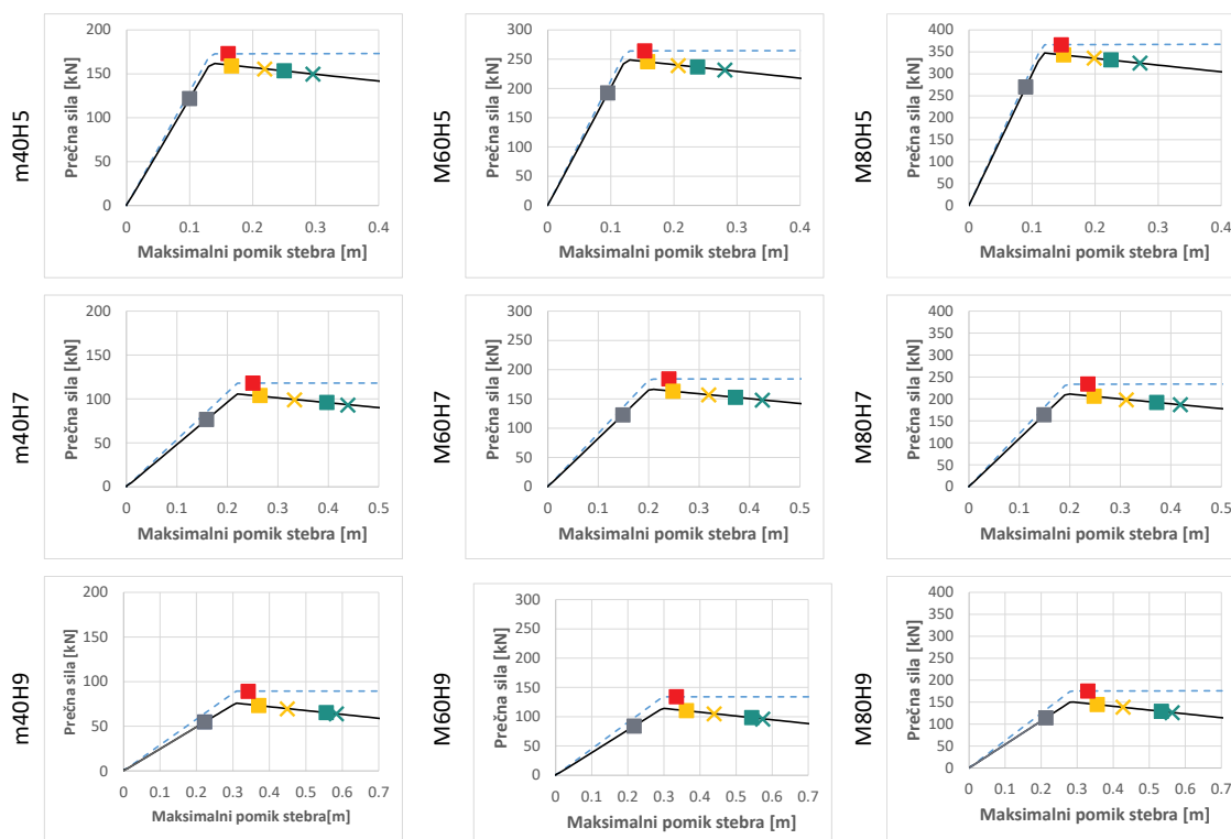
Legenda. Zahteve: ■ DL, ■ SD, ■ NC, ■ P-Δ zanemarjeno. Kapaciteta: X SD, X NC
