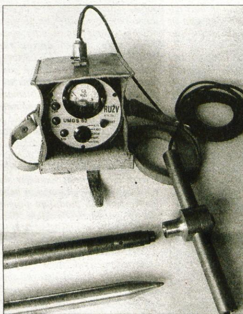
Uranova ruda je bila praviloma neločljiva od jalovine. Zato je bila nujna sistematska uporaba merilnikov radioaktivnosti. Na RUŽV se je uporabljalo več kot 200 merilnikov. Pri raziskavah so se sprva uporabljali scintilacijski in Geiger-Muellerjevi števeci ameriške, kanadske, francoske in ruske proizvodnje. Kasneje smo jih nūdomestili s števeci lastne proizvodnje. Na sliki Merilnik UMGS 82 konstruktorja Petra Zajca s T-sondo za meritev kosovne rude.
