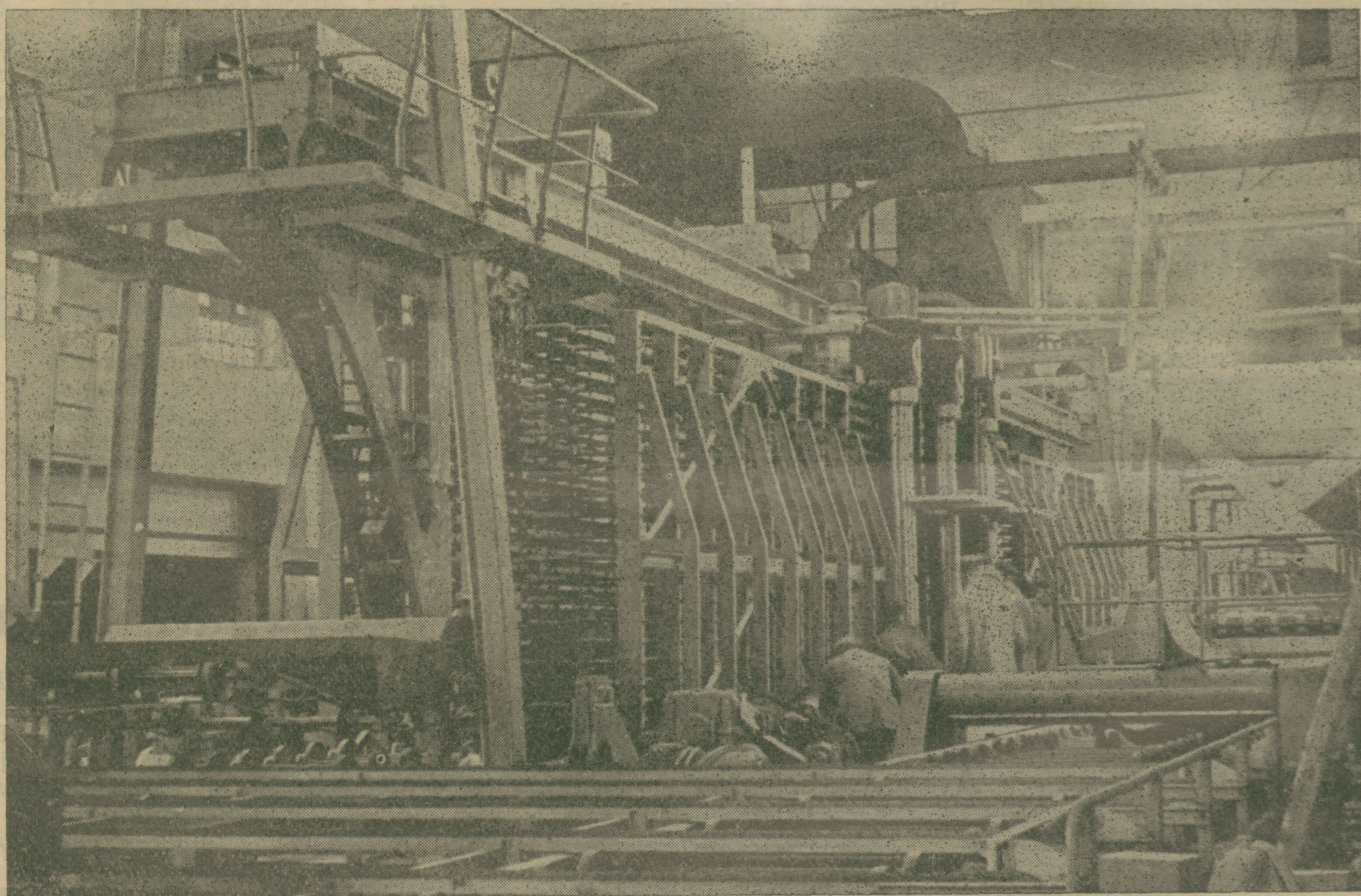
Rekonstrukcija obrata osnovne proizvodnje bo kmalu končana, le gola rebra strojev je treba še obdati s »kožo« — pločevino
