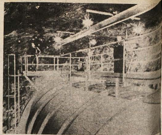
V zapuščenem rudniku zlata v Južni Dakoti poskušajo ugotoviti pretok nevtrinov z ogromno napravo. V hranilniku je več sto petklorotilena.
