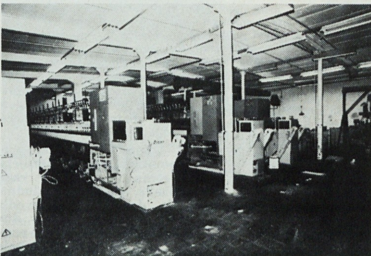
Oddelk predilnice 4 dobiva svojo končno podobo. Novi predilni prstanski stroji z avtomatskim snemanjem kopsov bodo v naslednjem mesecu pričeli poskusno obratovati.
