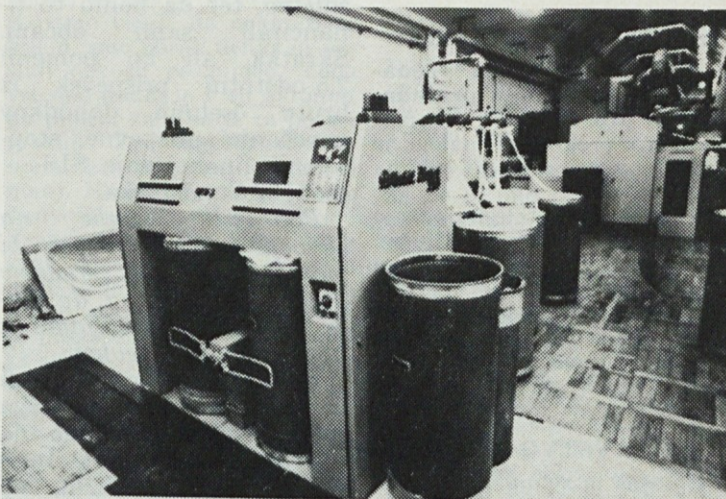
Postavili smo 4 nove raztezalko znamke Zinser-Krušik, za česano bombažno prejo. Dve že obratujeta, ostali dve pa čakata, da bo dokončana celotna česalna linija.
