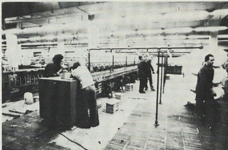
Montaža novih flyerjev znamke Krušik v oddelku sintetične. Stroj na sliki že obratuje.
