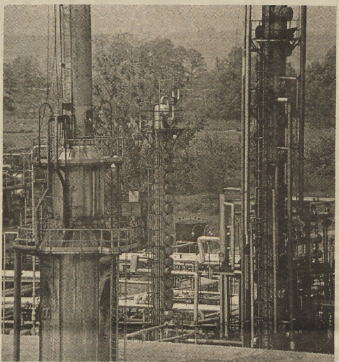
Peč in kolone za atmosfersko destilacijo nafte
