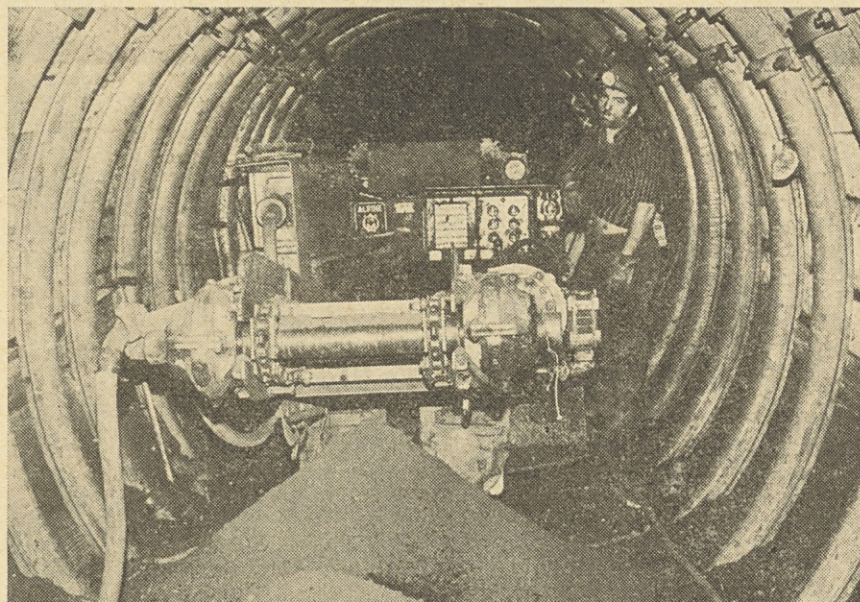
Jama Ojstro, kota 170. Preboj proge s strojem F6A. Terezija II polje. Ob stroju Anton Volavšek. (Foto: J. Kirič)
