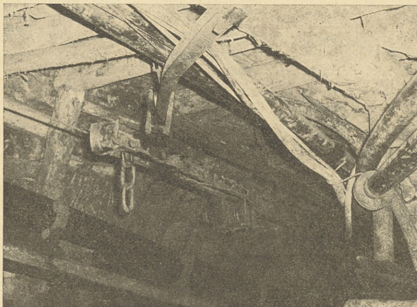
Viseča žičnica »Monorial« v jami Dol, vpadnik 193/163.
