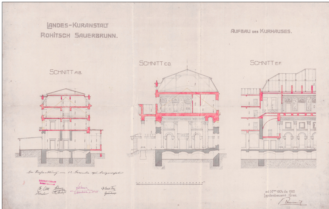
5. Načrt dvorane Zdraviliškega doma v Rogaschi Slatini, 1910, Zgodovinski arhiv Celje (© Zgodovinski arhiv Celje)
