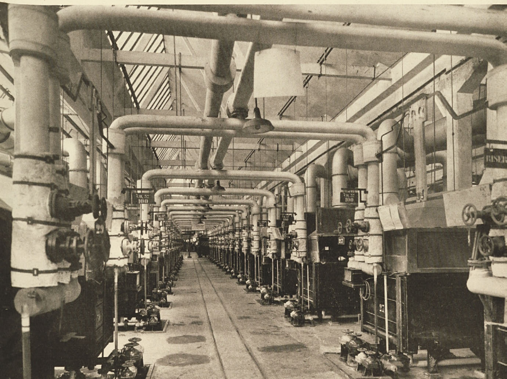
Ivrea-Chatillon - Impianto lavatura
