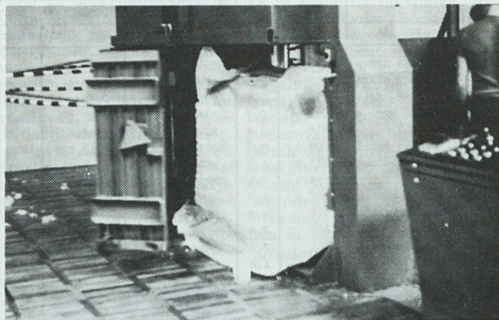
Stiskanje mešanic vlaken v bale
