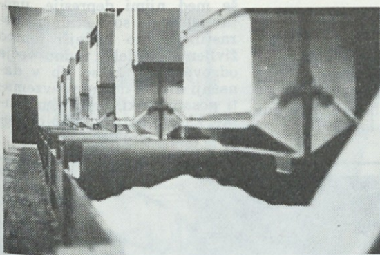
Novi in stari način melanžiranja
