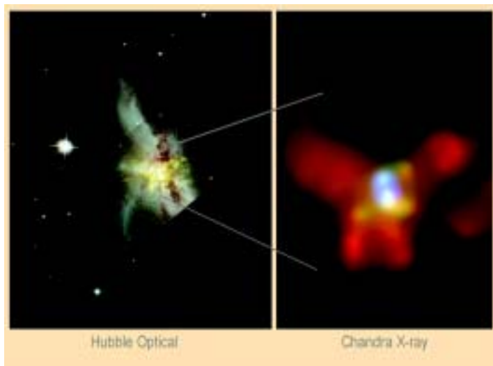
Galaksija, v katere središču se nahajata dve črni luknji, ki krožita druga okoli druge. Na levi je slika vesoljskega teleskopa Hubble, ki slika v vidni svetlobi, desno pa slika teleskopa Chandra, ki je posnela galaksijo v rentgenski svetlobi. Na desni sliki sta dobro vidna dva izvora rentgenskega sevanja, kar kaže na dve aktivni črni luknji.
