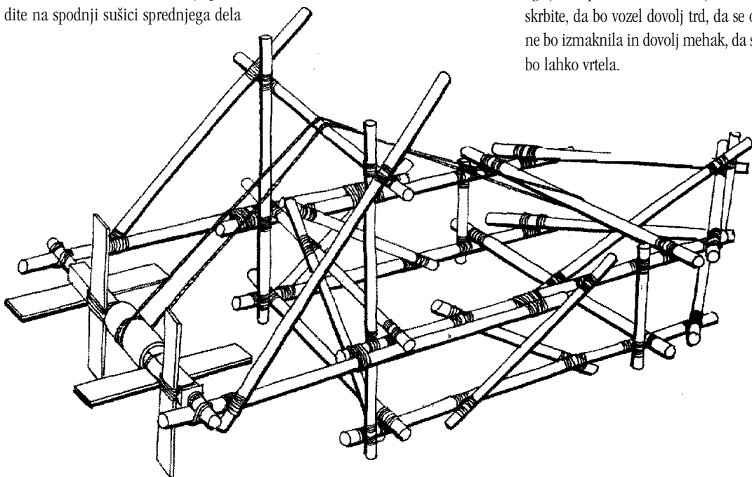
Okvir čolna in njegov pogon
