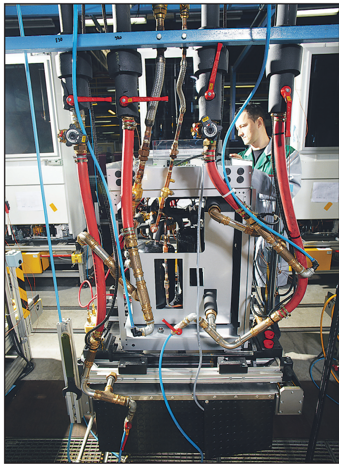
Iz proizvodnje toplotnih črpalk. Proizvajajo jih v obratu hladilno-zamrzovanih aparatov, kjer bodo jeseni začeli tudi proizvodnjo pomivalnih strojev.
