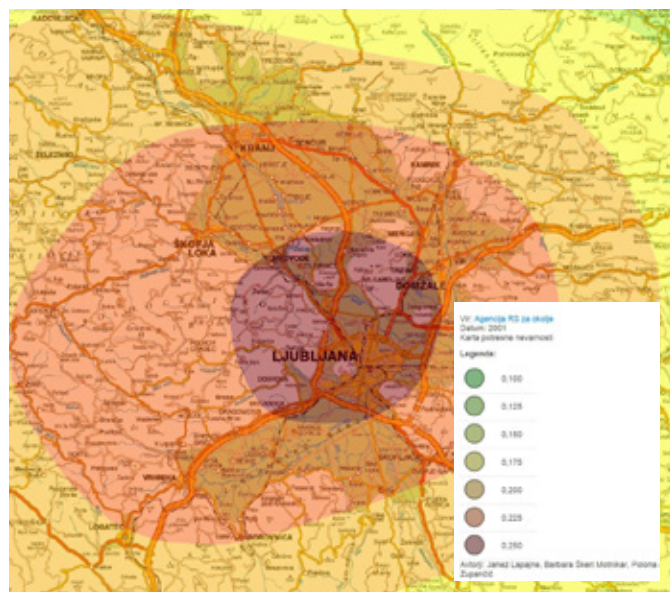
Karta potresnega pospeška tal za Slovenijo – izrez območja za osrednjo Slovenijo Vir: Geopedia, ARSO/Urad za seizmologijo in geologijo.
