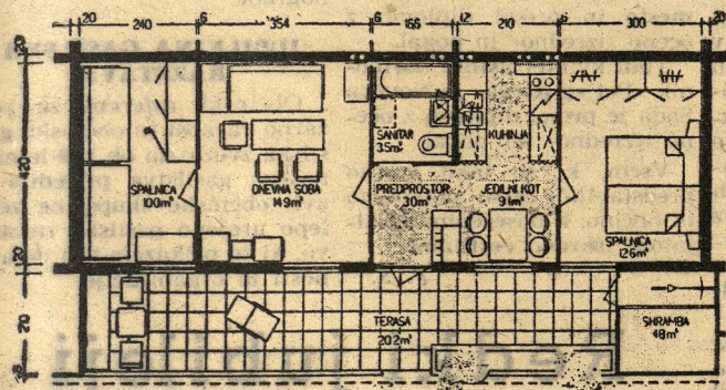
Tloris trosobnega stanovanja s skupno površino nekaj nad 78 kvadratnih metrov. Te hiše izdeluje in postavlja ljubljanski »Gradis« za — Koprčane
